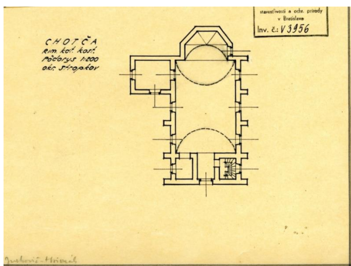
Pôdorys kamenného kostola z roku 1910 v mierke 1 : 200. Autor je architekt Dušan Jurkovič 395
